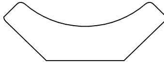
KL 304 .625 x 1.750
