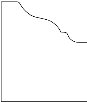
KL 310 1.750 x 1.500
