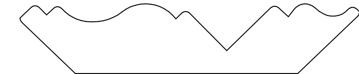
KL 341 .750 x 3.625
