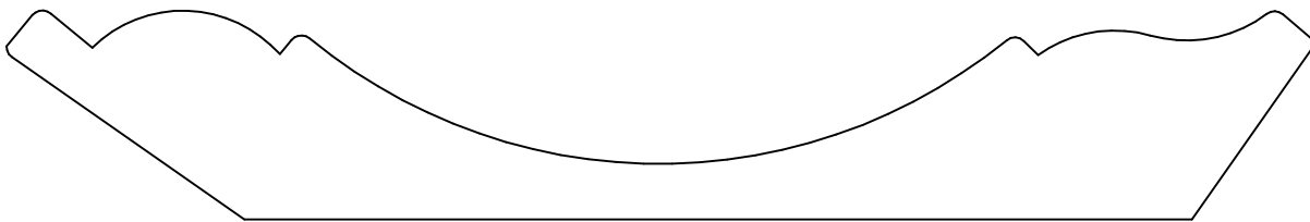
KL 1327 1.000 x 6.250
