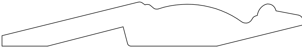
KL 3325 .812 x 5.500
