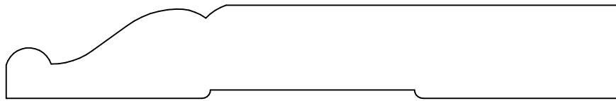
KL 1216 .687 x 4.500
