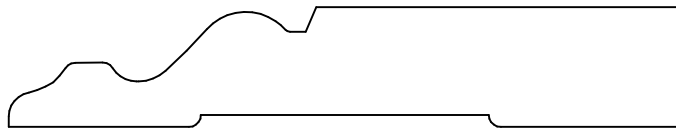
KL 4203 .625 x 3.500
