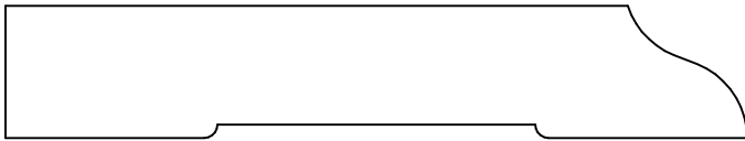
KL 214 .625 x 3.500
