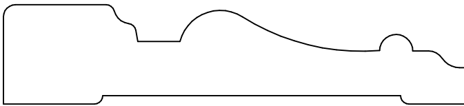
KL 4138 .750 x 3.500
